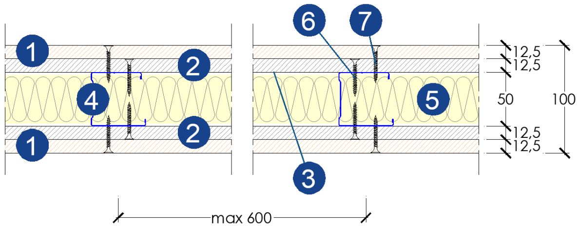
Figura 2_ Disegno tecnico: Sezione parte centrale (1)
