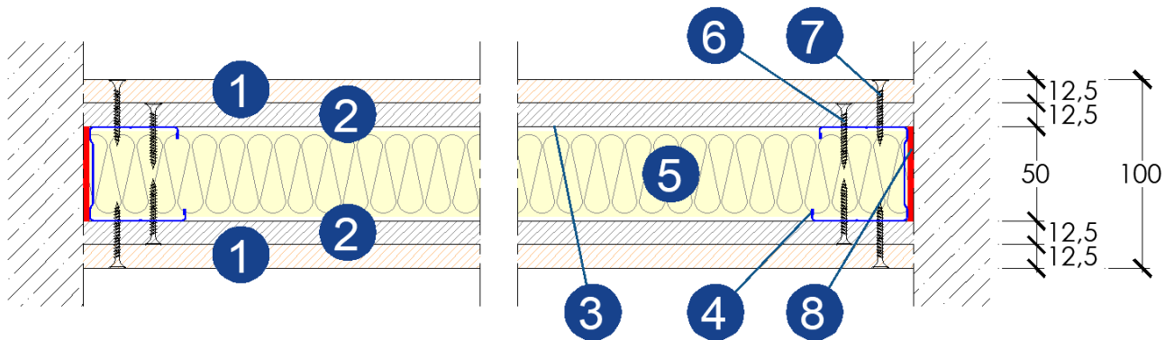
Figura 1_ Disegno tecnico: Sezione estremità (1)
