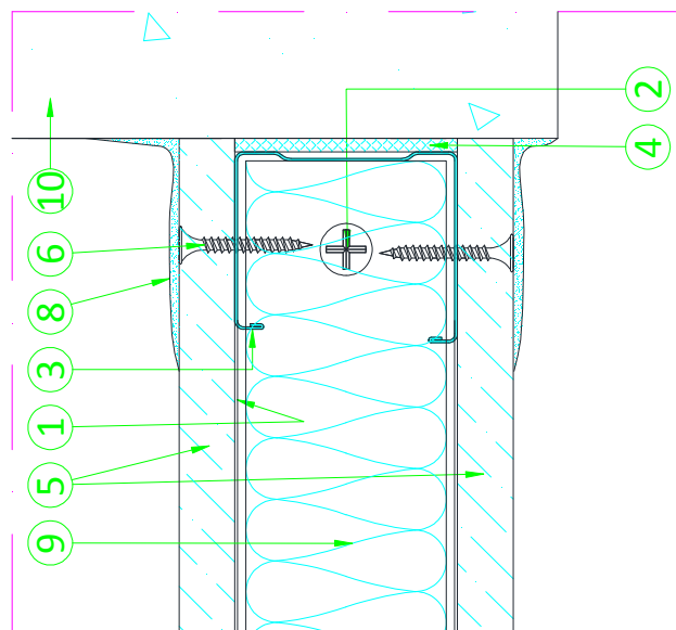
Particolare "B"
