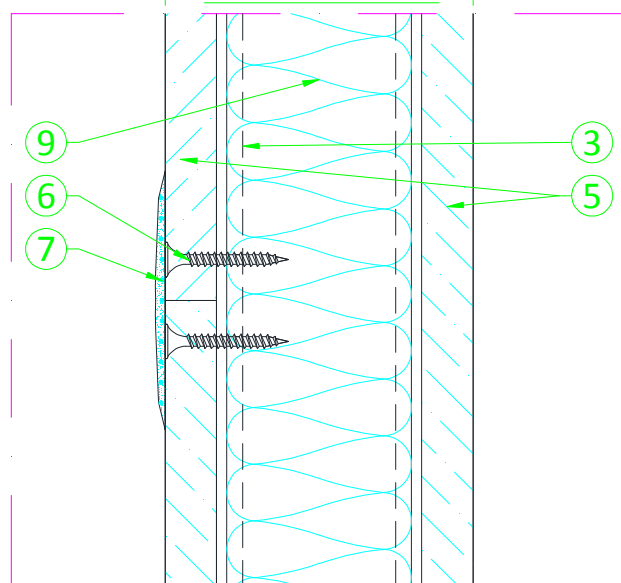
Particolare "D"
