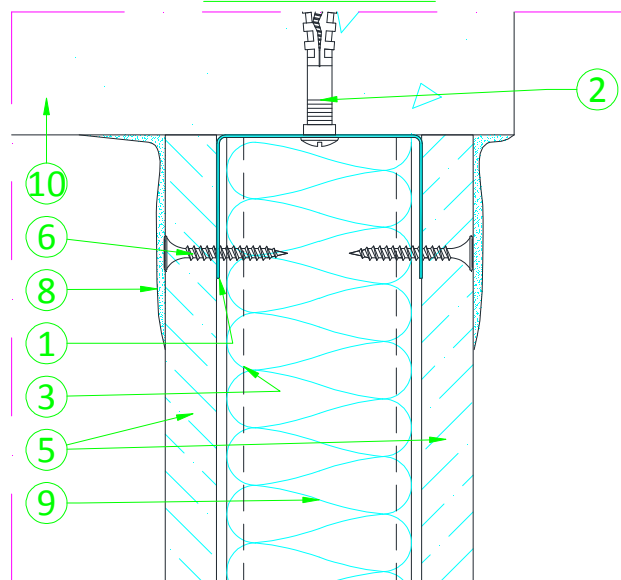
Particolare "C"
