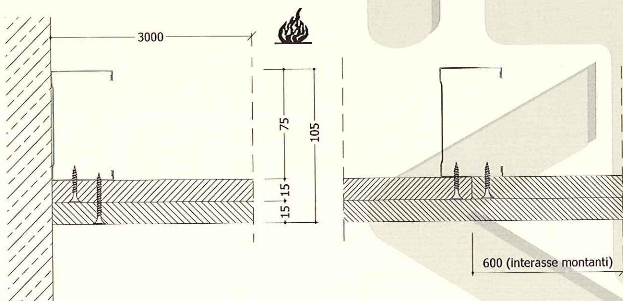
Sezione orizzontale campione in prova
