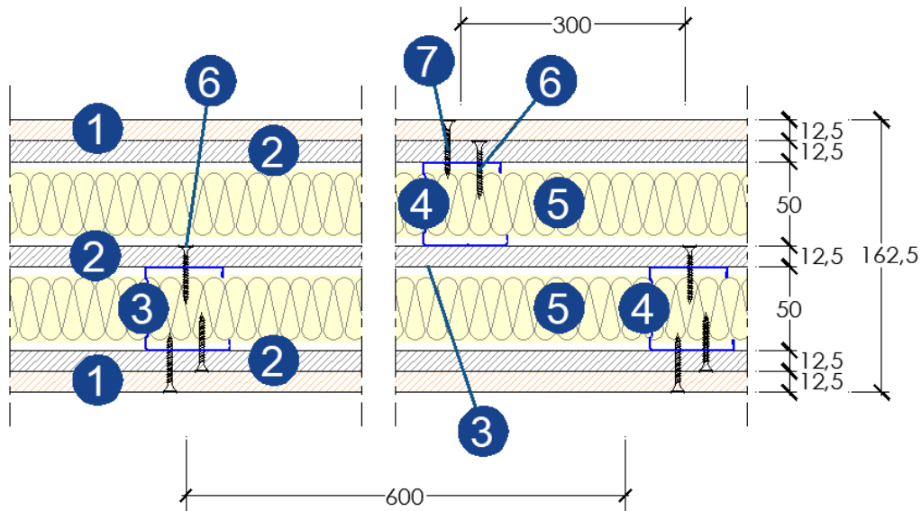
Figura 2_Disegno tecnico del campione: sezione - parte centrale (*)
