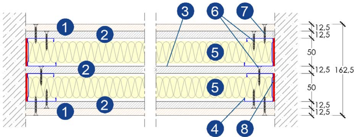
Figura 1_Disegno tecnico del campione: sezione - estremità (*)
