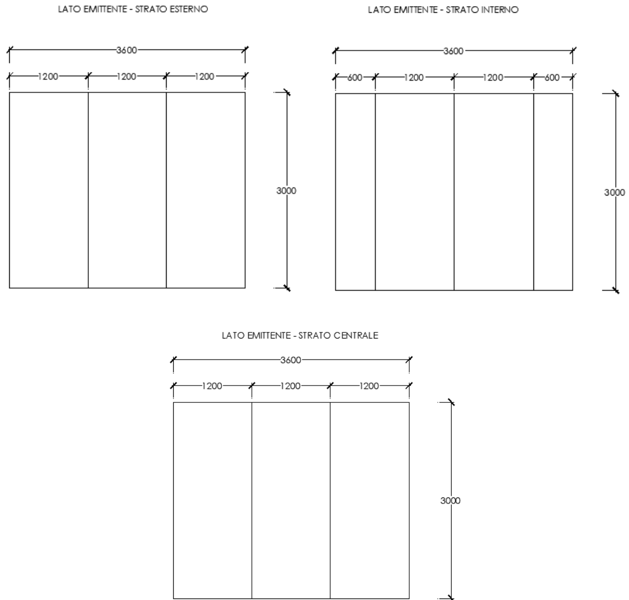
Figura 8_Prospetti lato camera emittente (*)
