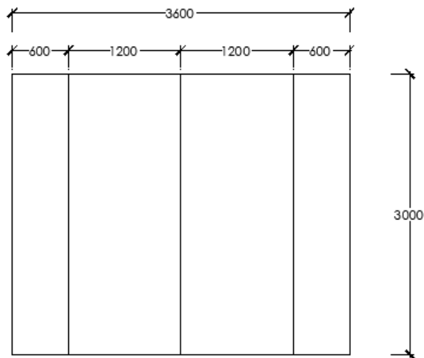
Figura 5_Prospetti lato camera ricevente (*)
