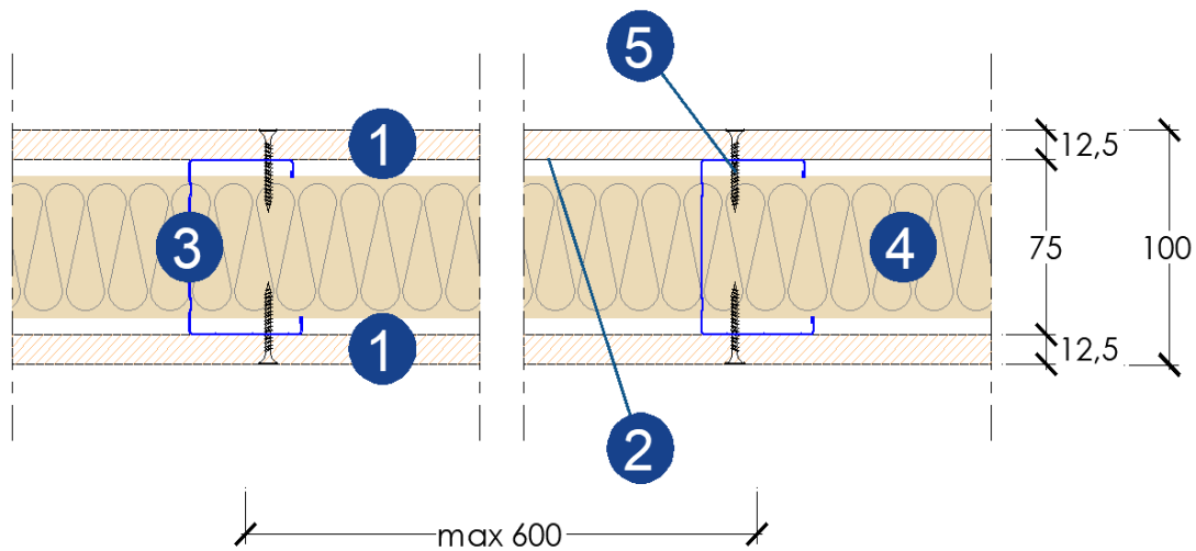
Figura 2_Disegno tecnico del campione: sezione – parte centrale (*)
