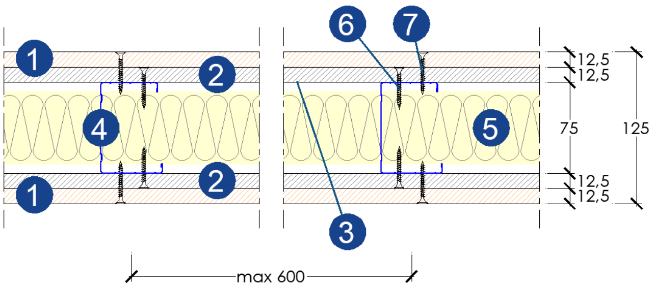
Figura 1_ Disegno tecnico: Sezione parte centrale (1)
