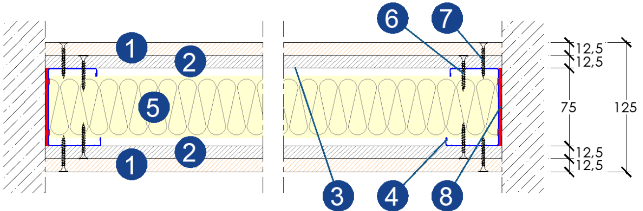
Figura 1_ Disegno tecnico: Sezione estremità (1)
