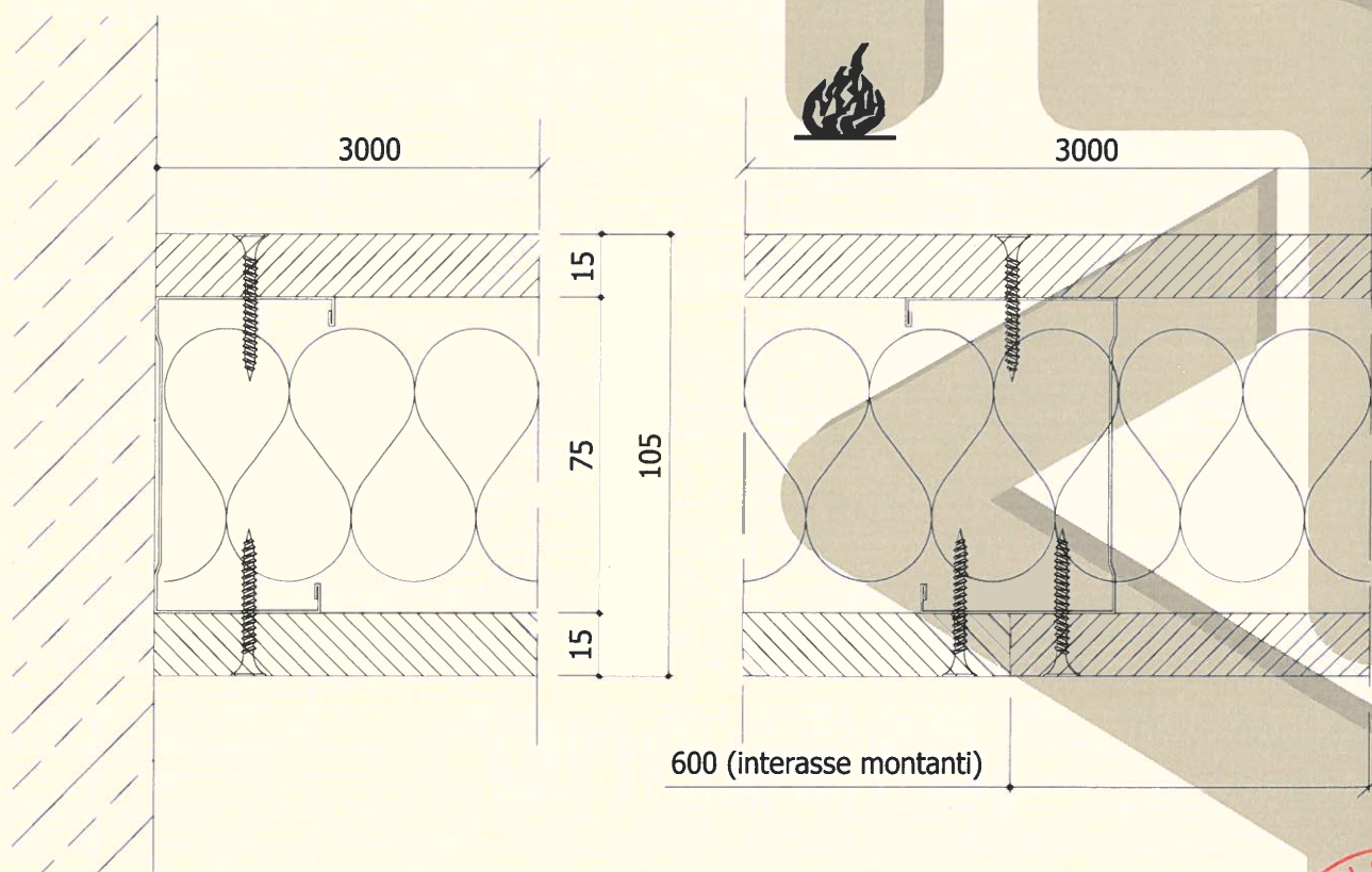
Sezione orizzontale del campione in prova
