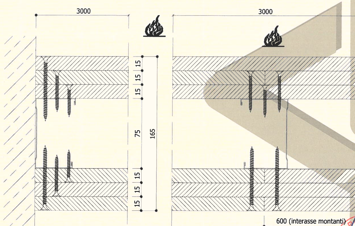
Sezione orizzontale del campione in prova
