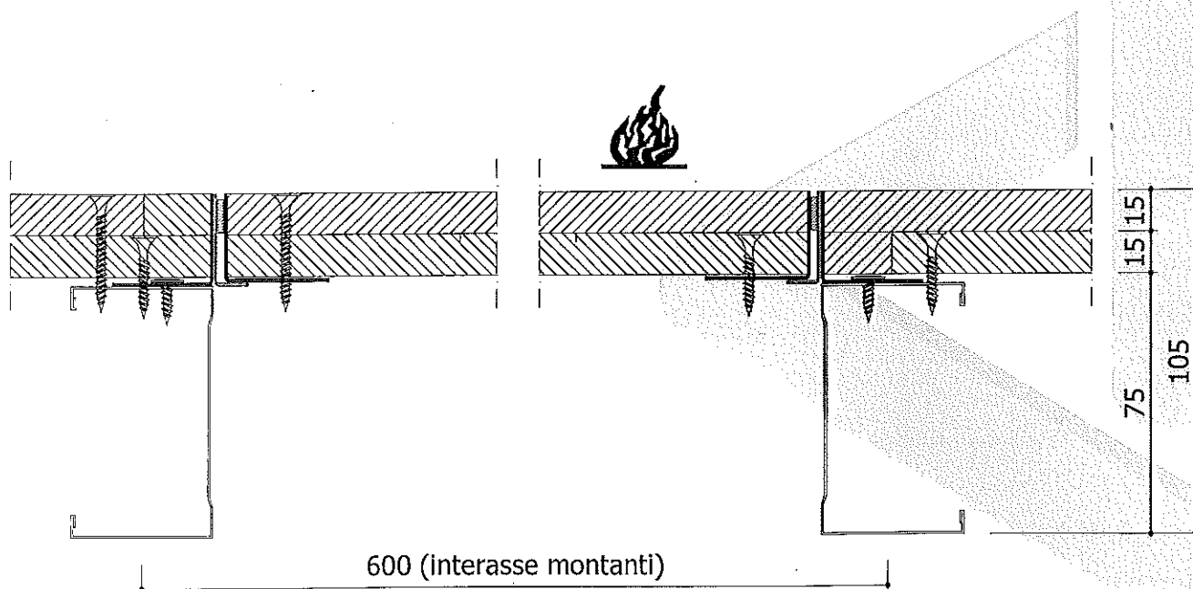
Particolare sezione orizzontale botola d'ispezione
