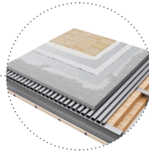
ILX SOL | TERRAZZA Copertura
