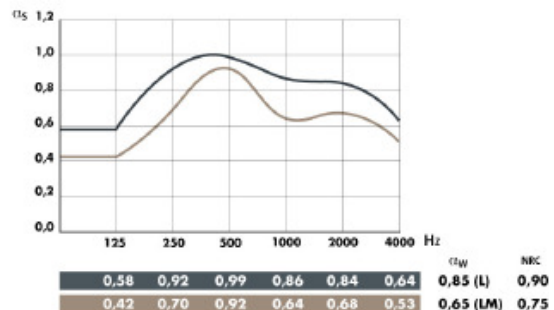
Coefficiente di assorbimento acustico \alpha_s
